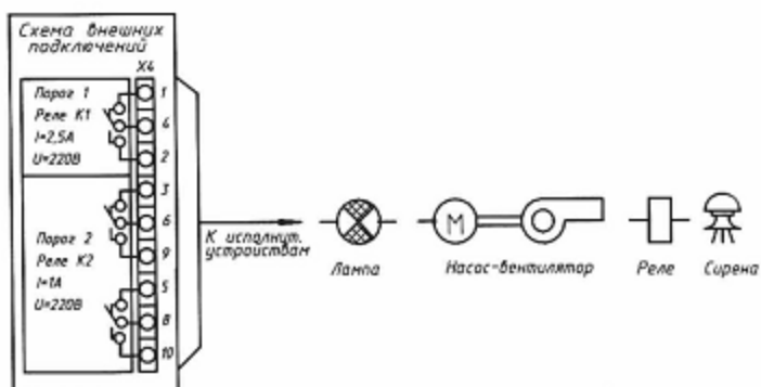
Схема внешних электрических соединений
